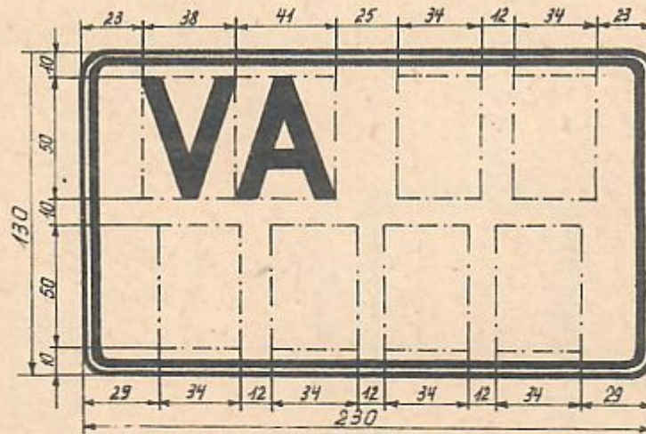
Bild 5 Kennzeichentafel (Form C) und Kennzeichen für Krafträder, P 601A, geländegängige Personenkraftwagen aus dem Import, Traktoren und handelsübliche Planierraupen
