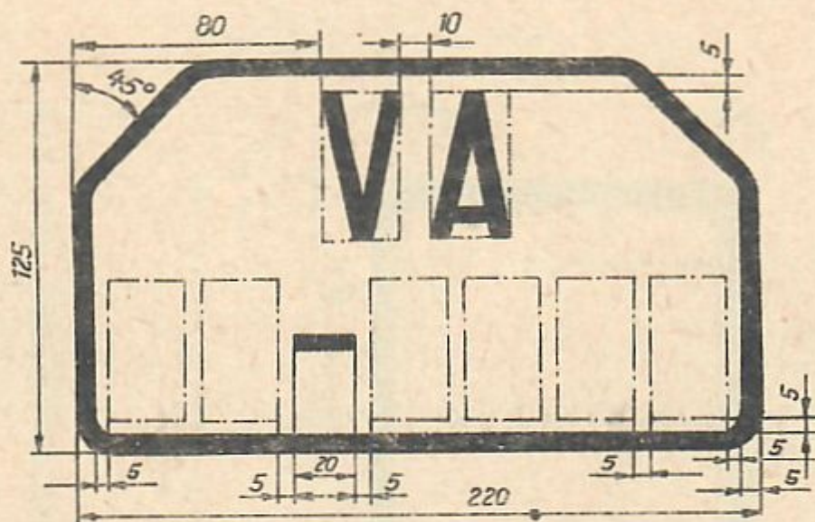
Bild 2 Kennzeichentafel und Kennzeichen für Krafträder, P 601A, geländegängige Personenkraftwagen aus dem Im- port, Traktoren und handelsübliche Planierraupen
