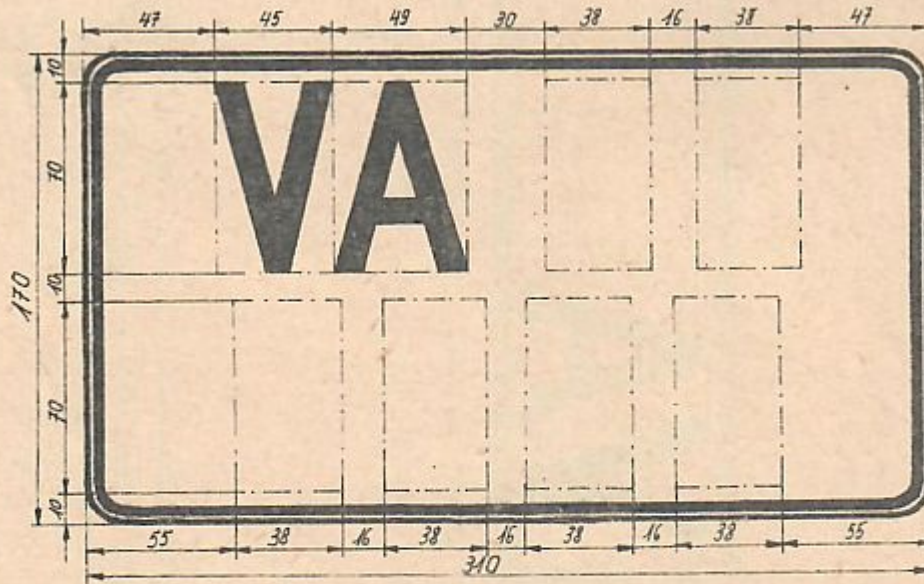
Bild 6 Kennzeichentafel (Form B) und Kennzeichen für gesondert festgelegte Kfz-Technik
