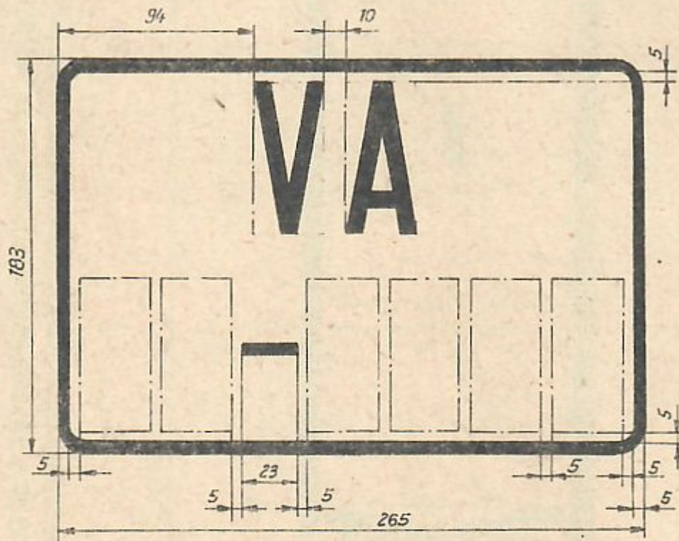
Bild 3 Kennzeichentafel und Kennzeichen für gesondert festgelegte Kfz-Technik
