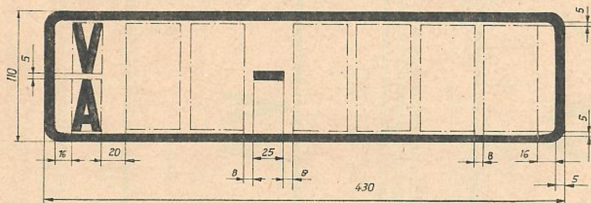
Bild 1 Kennzeichentafel und Kennzeichen für alle Typen und Arten der Kfz-Technik der NVA, mit Ausnahme der in den Bildern 2 und 3 aufgeführten Kfz-Technik
